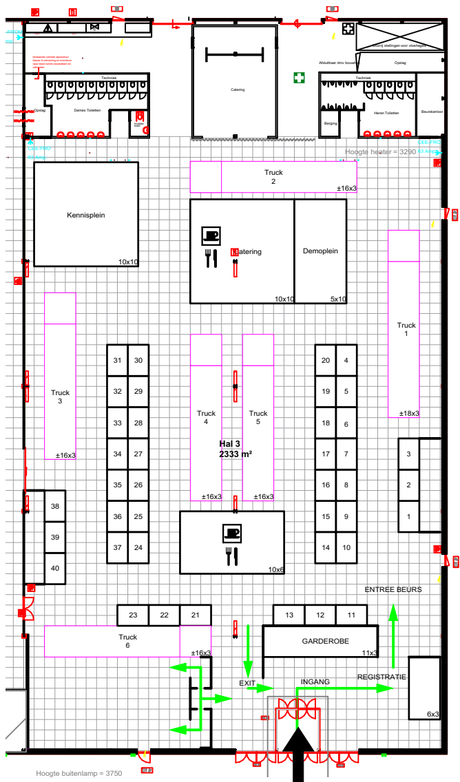
Plattegrond (1:500 A3)
